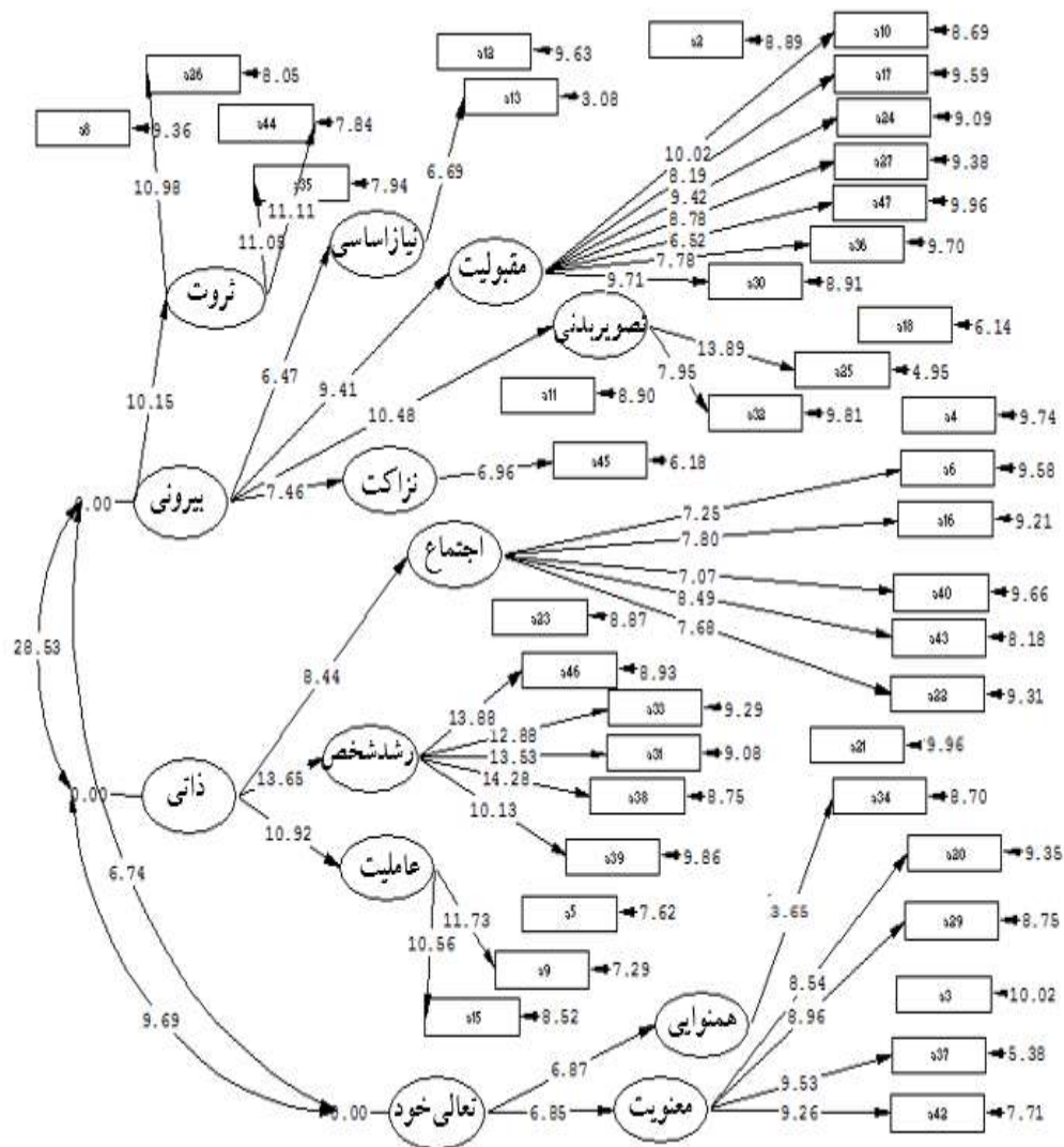
شکل ۴. الگو در حالت ضرایب معناداری
